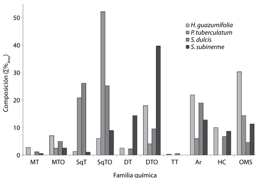
Fig. 1. Distribución de las familias químicas en los aceites esenciales de las hojas de las plantas (MT: monoterpenos, MTO: monoterpenos oxigenados, SqT: sesquiterpenos, SqTO: sesquiterpenos oxigenados, DT: diterpenos, DTO: diterpenos oxigenados, TT: triterpenos, Ar: derivados aromáticos, HC: hidrocarburos no terpenoidales, OMS: otros metabolitos secundarios no terpenoidales).
