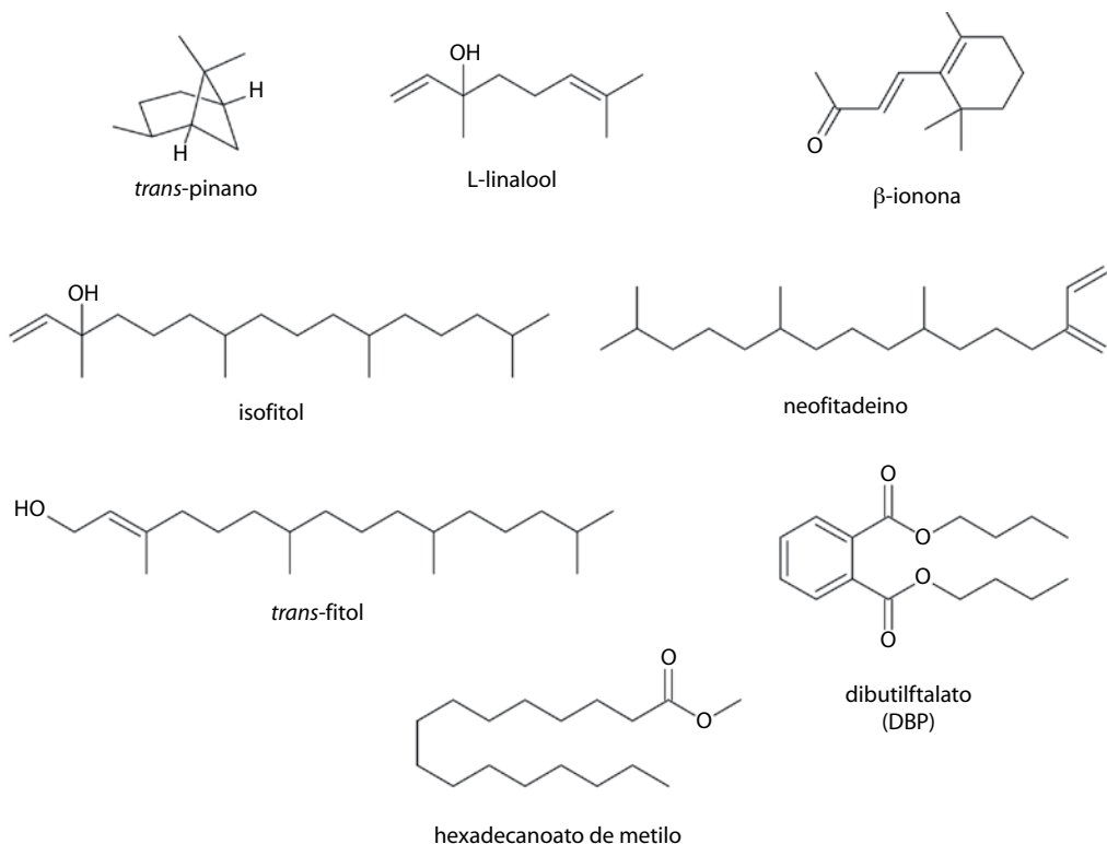
Fig. 2. Fórmula (representación) estructural de los metabolitos volátiles comunes en las esencias de tres de las especies estudiadas.
